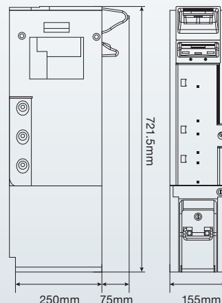
■ 外形図
