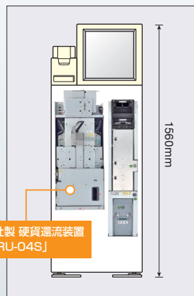
■ 透視図
